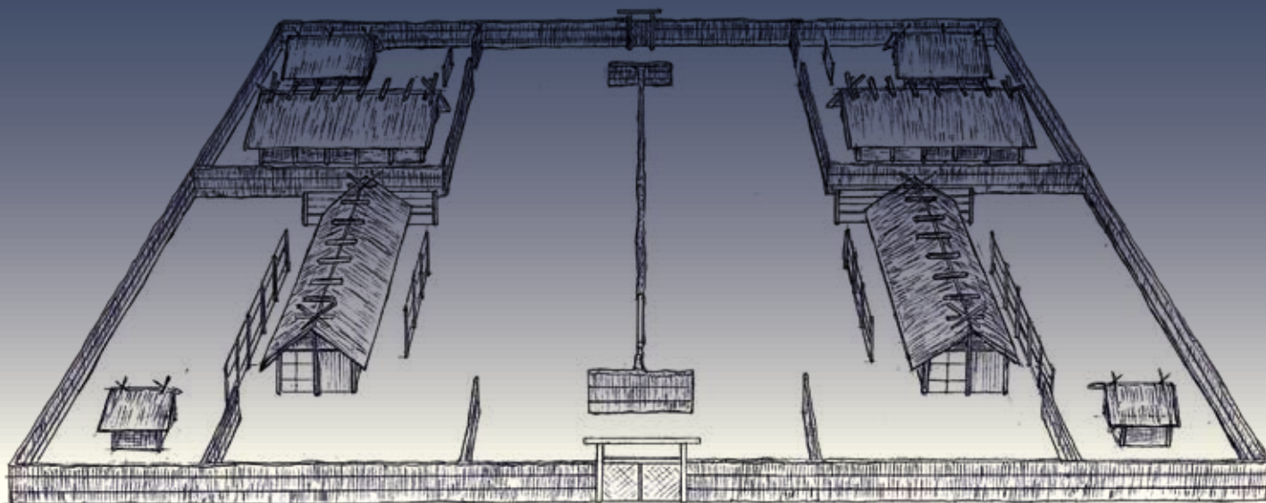
大嘗宮推定図(奈良時代)
